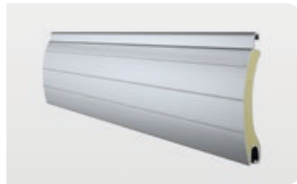
DT 500 Alu-Rollladenstab, ausgeschäumt, 49,80 x 11,20 mm
